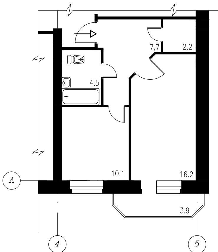
План объекта долевого строительства Однокомнатная квартира №35 S жилая = 16,20 м.кв., S общая = 44,60 м.кв.
