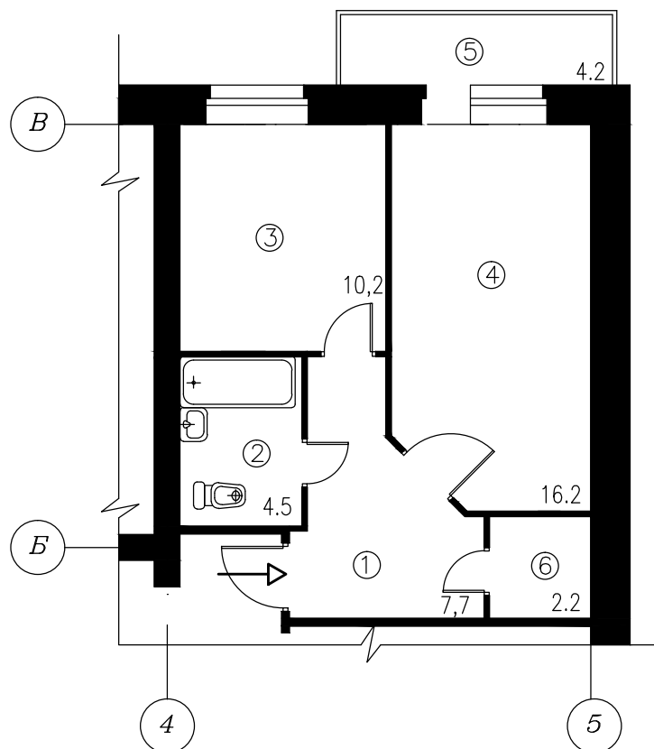
План объекта долевого строительства Однокомнатная квартира №34 S жилая = 16,20 м.кв., S общая = 45,00 м.кв.
