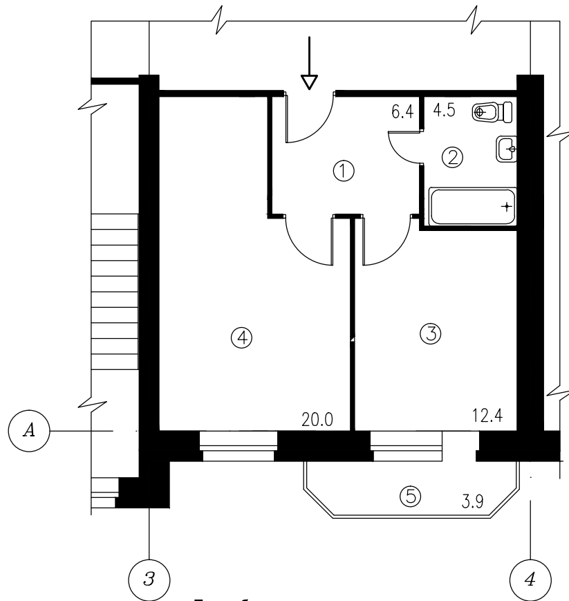
План объекта долевого строительства Однокомнатная квартира №11 S жилая = 20,00 м.кв., S общая = 47,20 м.кв.
