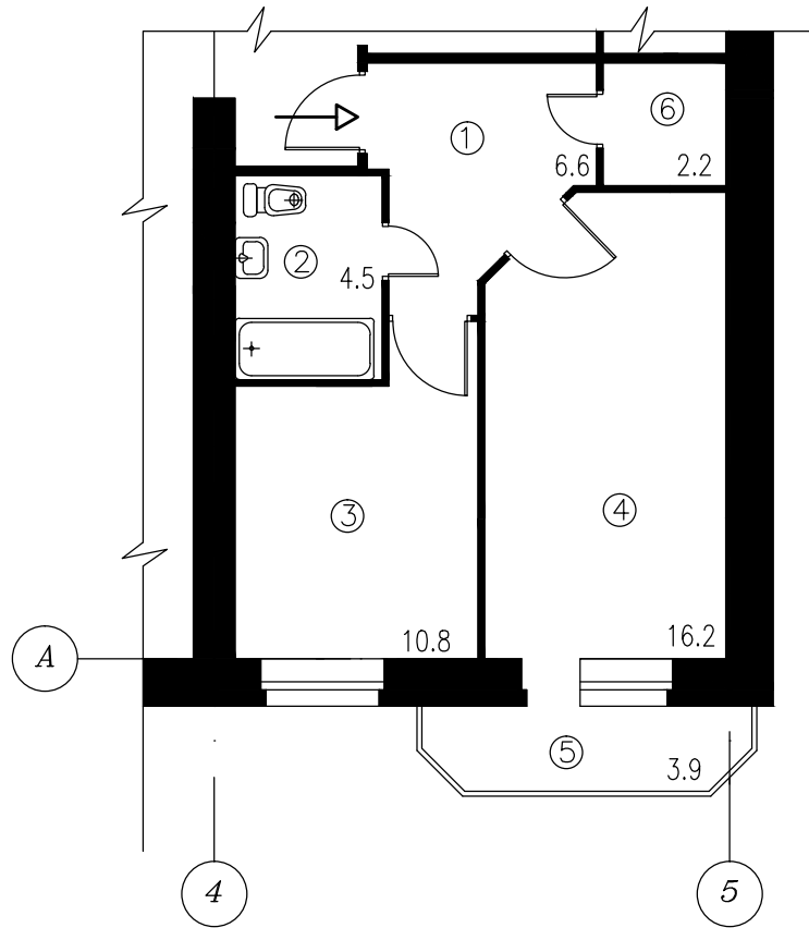
План объекта долевого строительства Однокомнатная квартира №10 S жилая = 16,20 м.кв., S общая = 44,20 м.кв.
